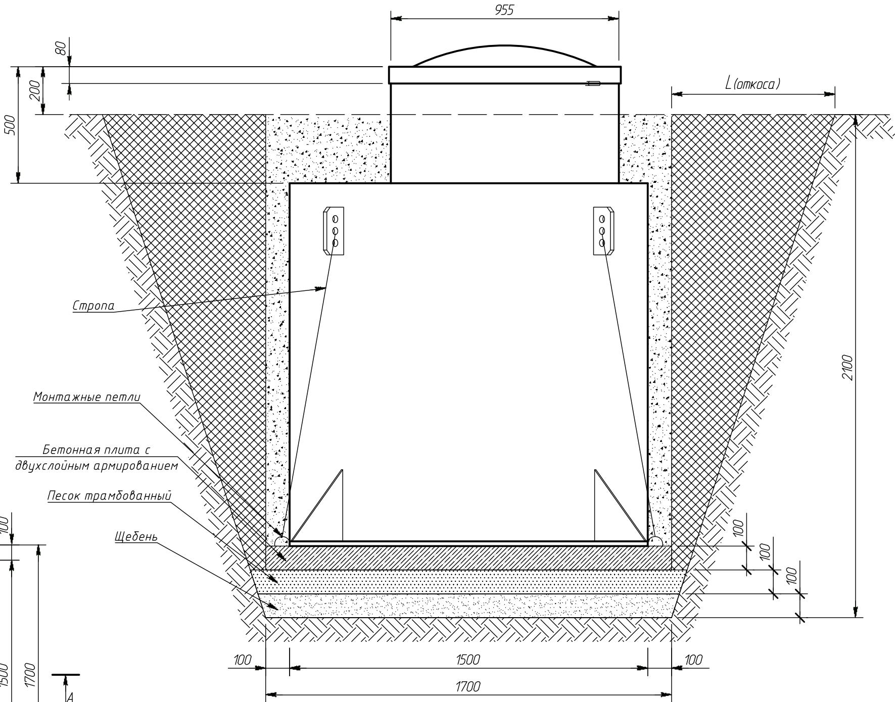
Разрез А-А М 1:16
